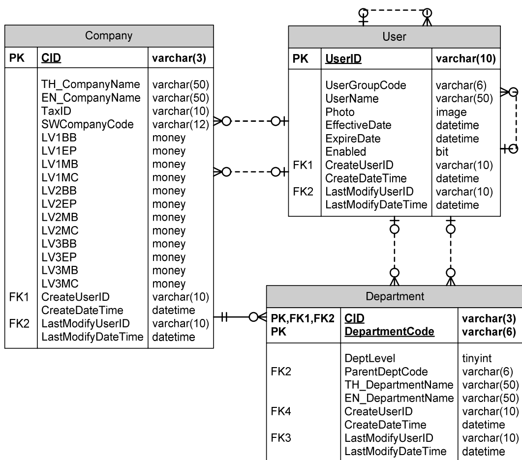
รูปที่ 7.4 แผนภาพ ER-Diagram ของกลุ่มข้อมูลฝ่าย
