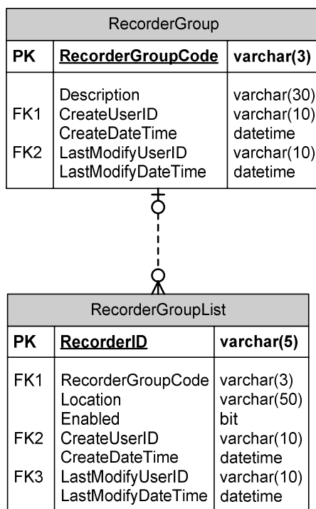
รูปที่ 7.15 แผนภาพ ER-Diagram ของกลุ่มข้อมูลเครื่องบันทึกเวลา
